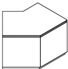
LD05 Corner 45° W1480 D1115 H760 mm
